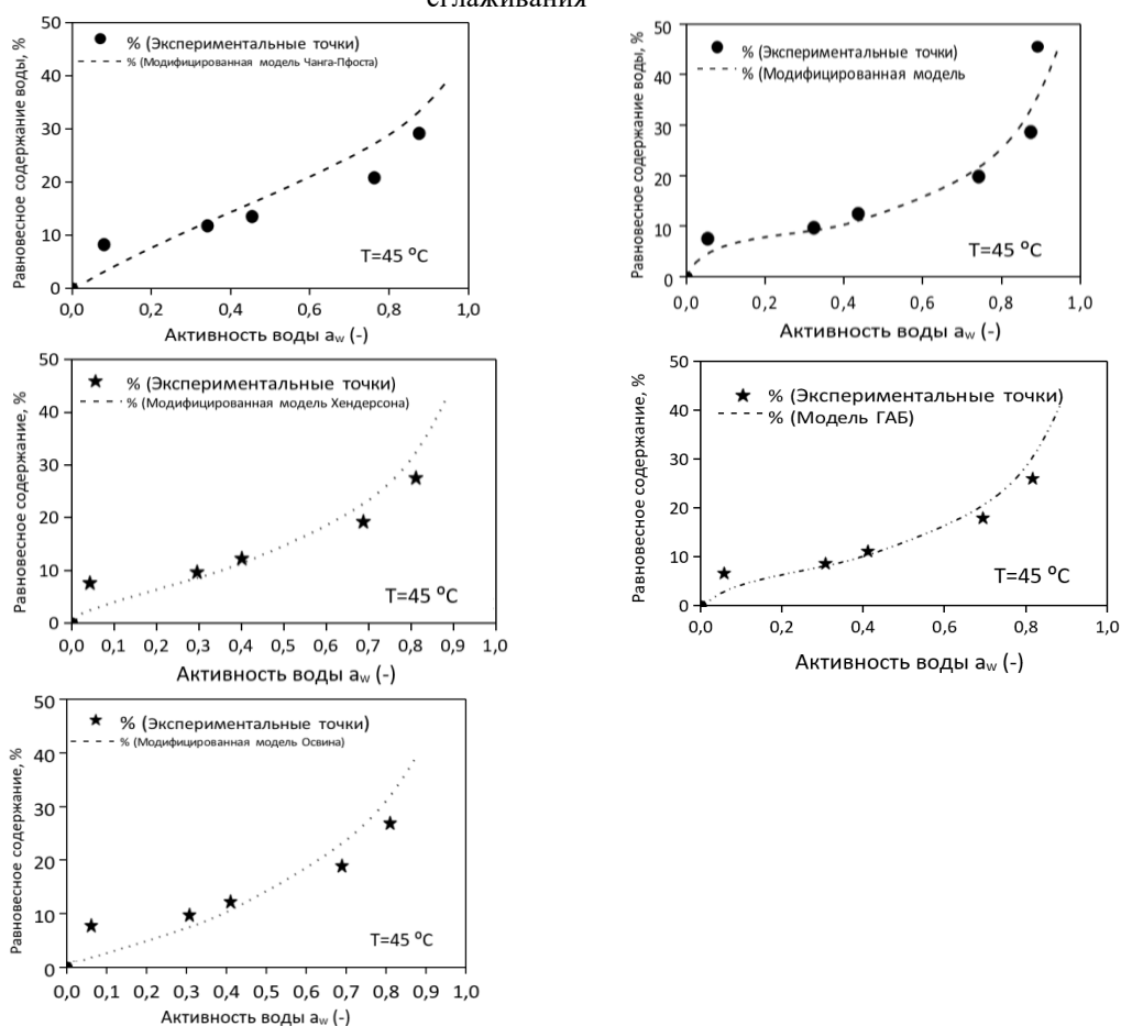
Рис. 2. Изотермы сорбции базилик обыкновенный ( Ocimum basilicum L. ), описанные пятью моделями сглаживания
