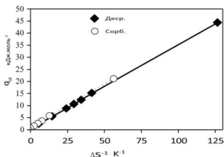
Рис. 5. Изменение энтальпии сорбции в зависимости от энтропии десорбции базилик обыкновенный ( Ocimum basilicum L.) (теория компенсации энтальпии/энтропии)
