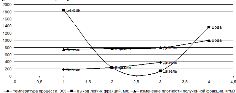
Súwret 3. Suyıltırılǵan neft shlamınan jeńil frakciyalardıń shıǵıwı hám payda bolǵan frakciyalardıń fizikalıq kórsetkishleriniń túrli temperaturalarda ózgeriwi (suyıltırıwshı-awır nafta)
