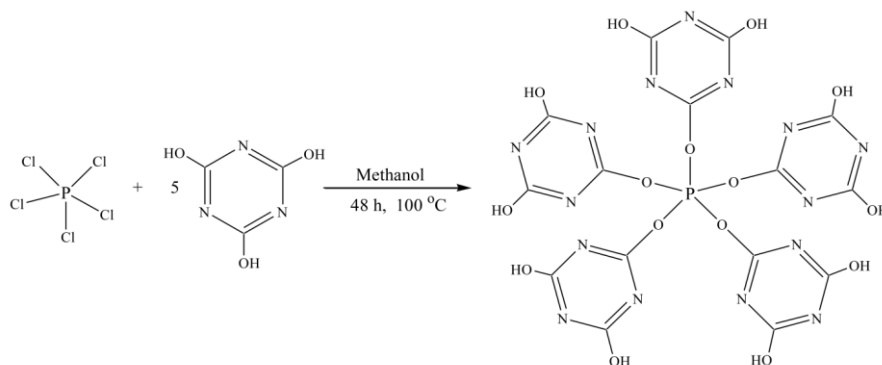
1-sxema. Quramında fosfor saqlaǵan oligomer PSK-1 sintezi.
