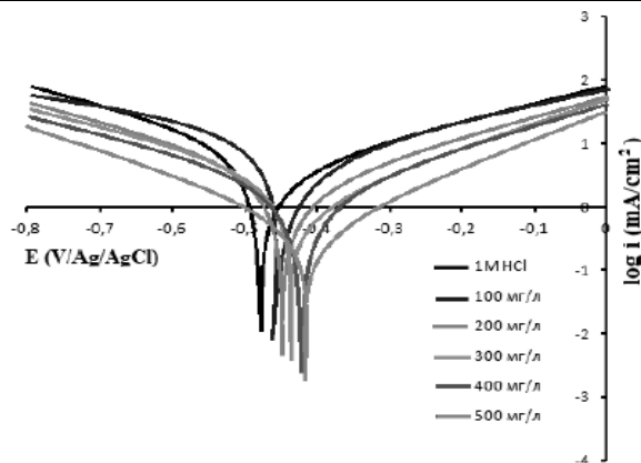
1-súwret. 298 K de PSK-1 diń hár túrli koncentraciyalarda ingibirlengen hám ingibirlenbegen 1M HCIda uglerodlı polattıń polarizaciya iymek sıyıqları.
