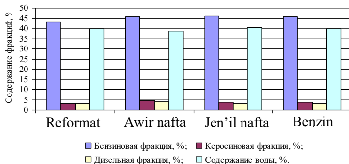
Сúwret 6. Neft shlamın hár túrli eritiwshiler menen suyıtırǵanda jeńil frakciyalardıń ajralıp shıǵıwı
