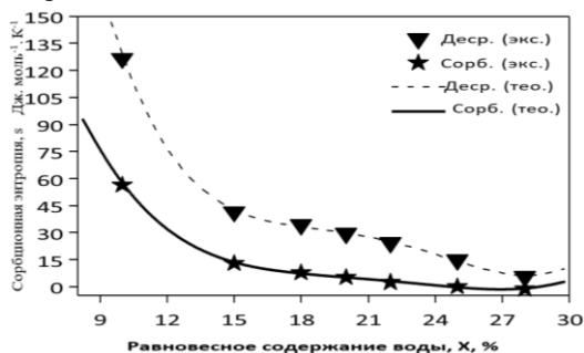
Рис. 4. Дифференциальная энтропия сорбции и десорбции базилик обыкновенный ( Ocimum basilicum L.) в зависимости от равновесного содержания воды
