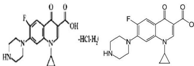
2- sxema. Siprofloksatsinni ajratib olish reaksiyasi
