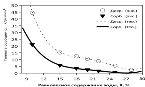
Рис. 3. Чистая изостерическая теплота сорбции и десорбции базилик обыкновенный ( Ocimum basilicum L.) в зависимости от равновесного содержания воды
