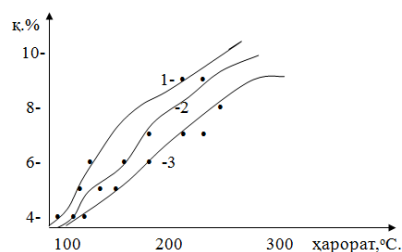
1-расм. Сув ва ФК билан поликонденсация жараёнида ҳосил бўлган антипиреннинг сувли эритмасини ёғочга шимилишини ўрганиш: 343 (3), 353 (2), 363 (1).
