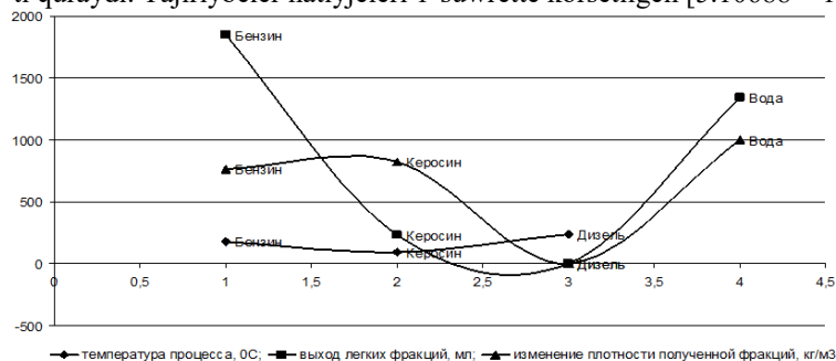
Súwret 1. Suyıltırılǵan neft shlamınan jeńil frakciyaların shıǵıwı hám payda bolǵan frakciyalardıń fizikalıq kórsetkishleriniń túrli temperaturalarda ózgeriwi (suyıltırıwshı-reformat)
