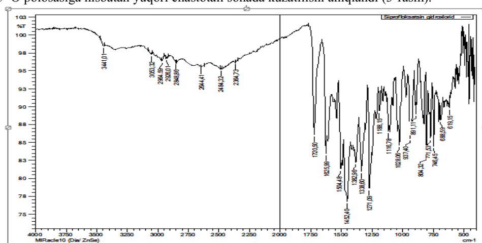
3- rasm. Siprofloksatsin molekulasi IQ- spektri
