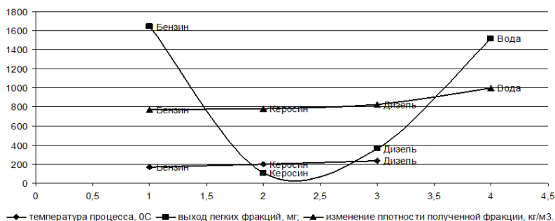
Súwret 2. Suyıltırılǵan neft shlamınan jeńil frakciyalardıń shıǵıwı hám payda bolǵan frakciyanıń fizikalıq kórsetkishleriniń túrli temperaturalarda ózgeriwi (suyıltırıwshı-jeńil nafta)
