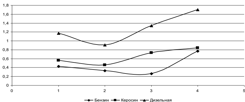
Сúwret 5. Alınǵan frakciyanıń 260^{\circ}\text{C} temperaturalarda kinematik jabısqaqlıǵınıń koefficienti
