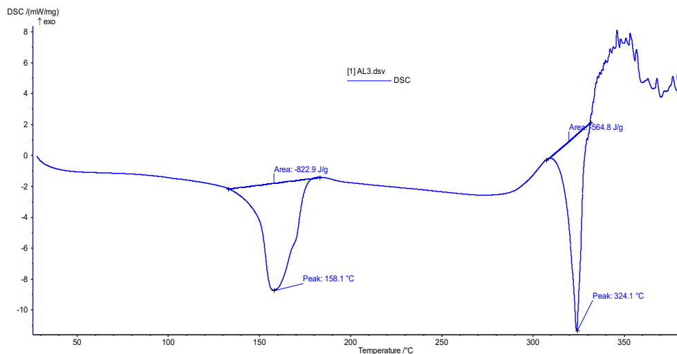
4- rasm. Siprofloksatsin molekulasi DSK
