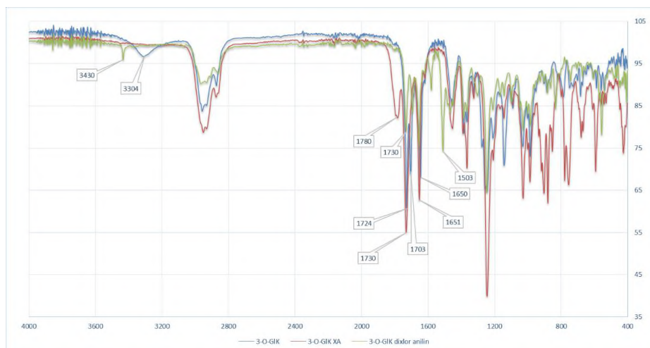
1-rasm. 3—atsetoksiglitsirret kislotasining 2,4-dixloranlin bilan olingan amidining IQ spektrlari
