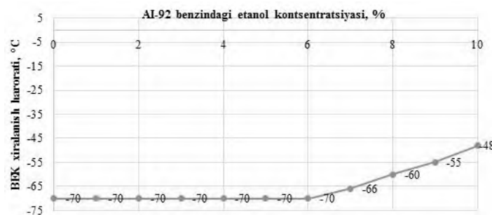
6-rasm. AI-92 benzinning 99 % li etanol bilan turli kontsentratsiyalardagi olingan BEKlarining xiralanish haroratlari
