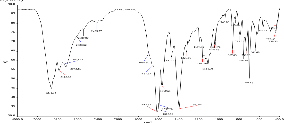
Рис.1. ИК-спектр поглощения смешанноамидного координационного соединения нитрата магния с карбамидом и тиокарбамидом состава \text{Mg}(\text{NO}_3)_2 \cdot \text{HCONH}_2 \cdot \text{CS}(\text{NH}_2)_2 \cdot \text{H}_2\text{O}
