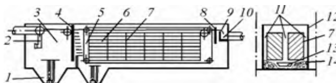
Рисунок 3. Многоярусный отстойник нефтеловушки с перекрестным движением рабочего потока жидкости и выделенного осадка из нефти: 1 - приямок для осадка; 2 - впускное устройство; 3 - зона грубой очистки; 4 - распределительное устройство; 5 - зона тонкой очистки; 6 - ярусы; 7 – блок пластин; 8 - полупогруженная перегородка; 9 - водослив; 10 - водоприемный лоток; 11 - зазоры, перегораживаемые щитками; 12 - корпус; 13 - скребок; 14 - лоток
