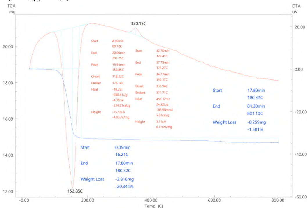
3 rasm. Ustyurt 2 gips konining termik tahlil grafigi
