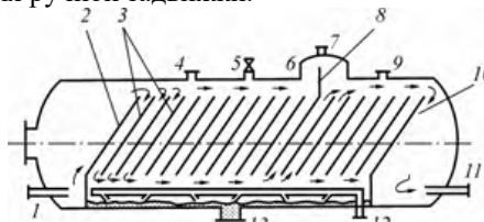
Рисунок 2. Схема многоярусного тонкослойного отстойника для очистки сточных вод: 1 - патрубок ввода сточной воды; 2, 8 и 10 - перегородки; 3 - пластина; 4 - штуцер для выпуска воздуха; 5 - предохранительный клапан; 6 - нефтесборник; 7 - штуцер для выпуска уловленных нефтепродуктов; 9 - штуцер вакуум-клапана; 11 - штуцер для вывода осветленной воды; 12 - труба для смыва осадка; 13 - штуцер для вывода шлама.
