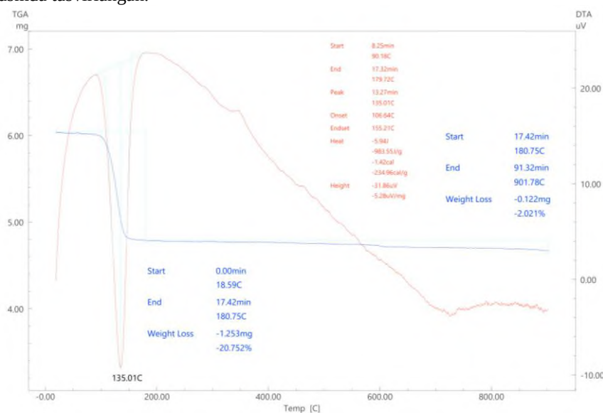
2 rasm. Ustyurt 1 gips konining termik tahlil grafigi
