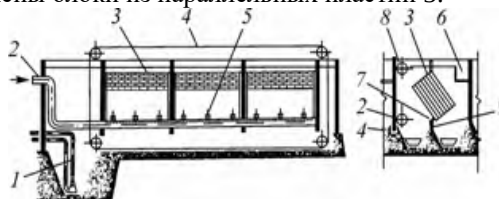
Рисунок 1. Схема тонкослойного отстойника нефтеловушки с противоточным движением воды и выделенной нефти: 1 - гидрозлеватор для удаления осадка; 2 - заглубленный трубопровод для подачи загрязненной жидкости; 3 - параллельные пластины; 4 - скребковый транспортер; 5 - насадки; 6 - лоток для приема очищенной жидкости; 7 - шарнирное соединение; 8 - нефтесборная труба; 9 - перегородка
