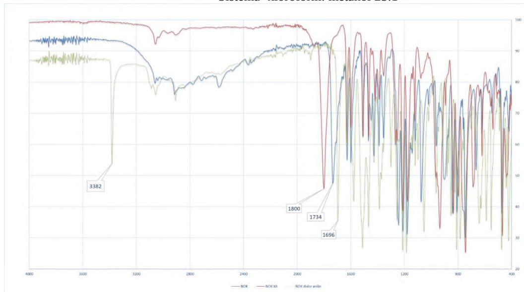
3-rasm. Naftoksi sirka kislotasining 2,4-dixloranlin bilan olingan amidining IQ spektrlari
