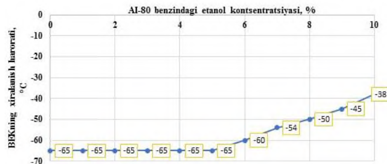
5-rasm. AI-80 benzinning 99 % li etanol bilan turli kontsentratsiyalardagi olingan BEKlarining xiralanish haroratlari
