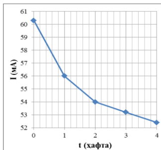
1-расм. Қуёш элементи қисқа туташув токи- I_{кт} нинг биринчи ойдаги ўзгариш графиги
