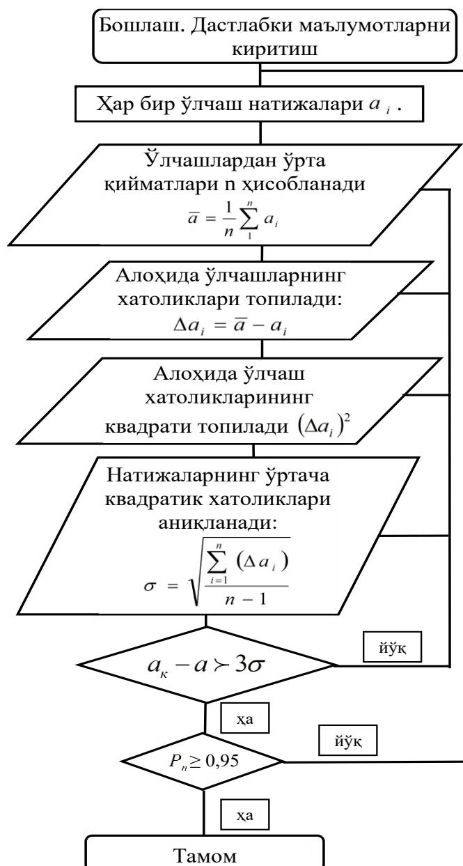
3 - расм. Пахта-тўқимачилик кластери корхонасининг энергетик кўрсаткичларини ҳисоблаш алгоритми
