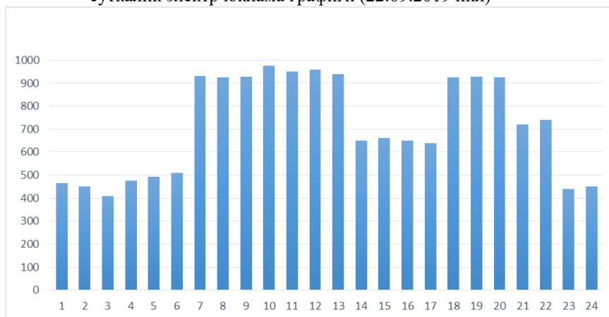
2 - расм. “WBM ROMITEX” МЧЖ пахта-тўқимачилик кластери корхонасининг пахта тозалаш заводининг суткалик электр юклама графиги (22.09.2019 йил)
