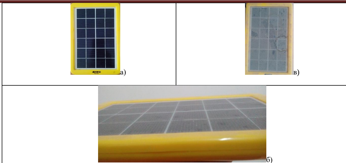
3-расм. Тажриба ўтказилаётган қуёш элементининг дастлабки ҳолати- (а), уч ойдан кейинги ҳолати- (б) ва бир йилдан кейинги ҳолати-(в)
