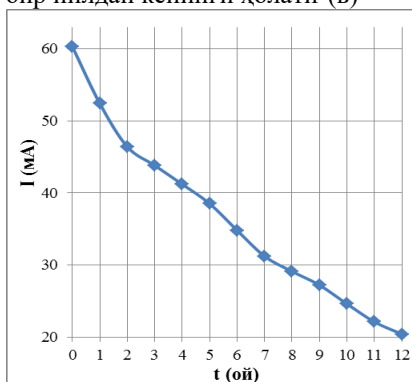
4-расм. Қисқа туташув токи- ( I_{кт} ) қийматининг ҳар бир ойга- (t) мос равишда ўзгарганлик графиги
