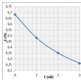
2-расм. Қуёш элементи параметрлари ( I_{кт} ва V_{с\text{ю}} )нинг уч ой давомида ўзгариш графиги
