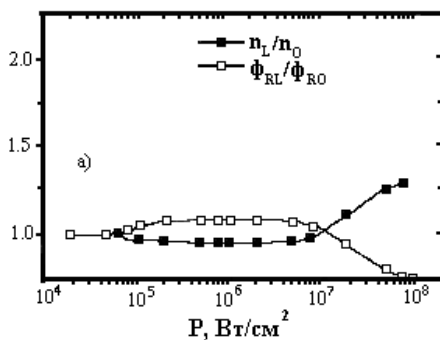
3a-súwret. W-n-GaAs Shottki barerliyarımótkizgishli diodlardıń tiykarǵı parametrleri - barer biyikliginiń n_L/n_0 ideallıq koefficientiniń dozalıq ǵárezziligi.
