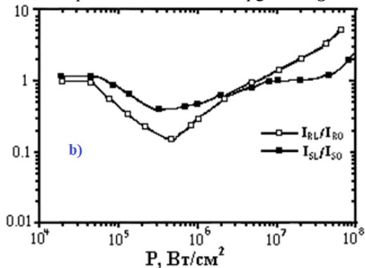
3b-súwret. W-n-GaAs Shottki barerliyarımótkizgishli diodlardıń tiykarǵı parametrleri - I_{SL}/I_{SO} toyınıw togınıń hám 2V kernewde ólshengen I_{RL}/I_{RO} keritoktıń dozalıq ǵárezziligi.
