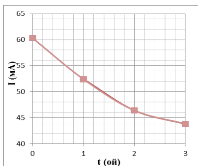
2-расм. Қуёш элементи параметрлари ( I_{кт} ва V_{с\text{ю}} )нинг уч ой давомида ўзгариш графиги
