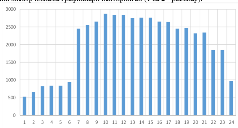
1 - расм. “WBM ROMITEX” МЧЖ пахта-тўқимачилик кластери корхонасининг текстил комбинатининг суткалик электр юклама графиги (22.09.2019 йил)
