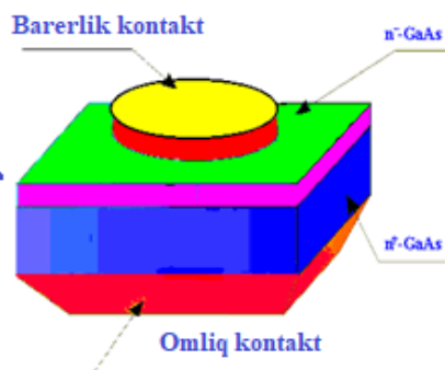
2-súwret. Metall-arsenid galliy kontaktınıń dúzilisi
