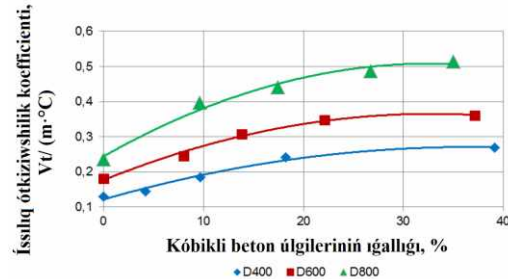
2-сúwрет. Микрокремнезюм тийкарındaǵı автоклав болмаǵан кóbикбетонларdıń ıssılıq ótkiziwsheńlik koefficientleriniń olardıń ıǵallıǵına baylanıslılıǵı
