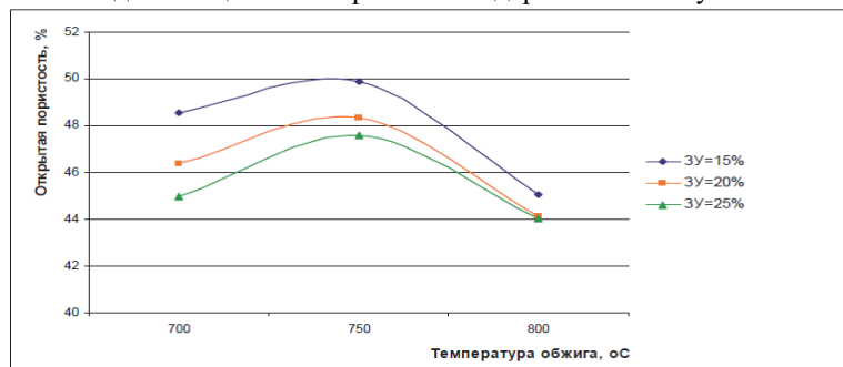
Рис. 3. Зависимость открытой пористости от содержания золы-уноса и температуры обжига
