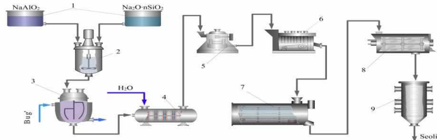
3-rasm. Seolit ishlab chiqarish texnologik sxemasi.
