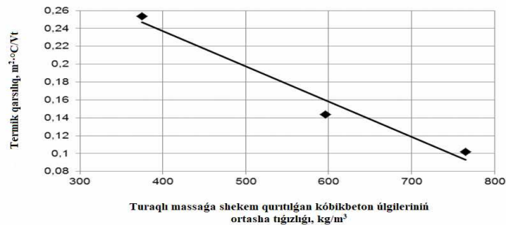
4-súwret. Mikrokremnezyom tiykarındaǵı avtoklav bolmaǵan kóbikbetonnıń termik qarsılıǵınıń onıń ortasha tıgızlıǵına baylanıslılıǵı
