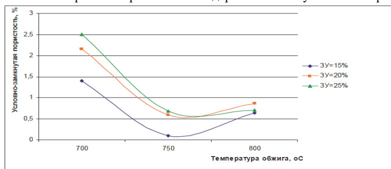
Рис. 4. Зависимость условно-замкнутой пористости от содержания золы-уноса и температуры обжига
