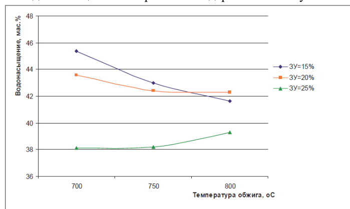
Рис. 2. Зависимость водонасыщения материала от содержания золы-уноса и температуры обжига
