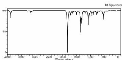
2-rasm. 1,3-Dimetil-5(6)-benzoilbenzimidazolin-2-onning IQ-spektri
