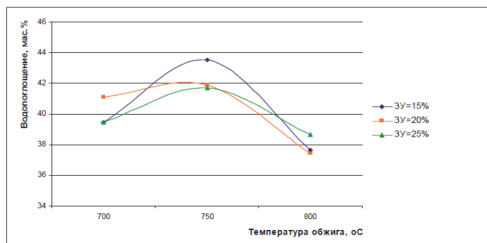
Рис. 1. Зависимость водопоглощения материала от содержания золы-уноса и температуры обжига
