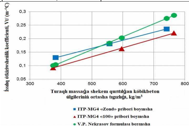
3-сúwрет. Микрокремнезюм тийкарındaǵı автоклав болмаǵан кóbикбетонnıń ıssılıq ótkiziwsheńlik koefficientleriniń ortasha tıǵızlıqqa baylanıslılıǵı
