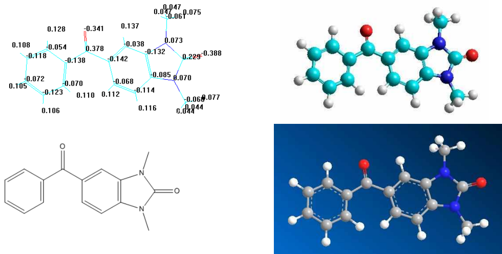
1-rasm. 1,3-Dimetil-5(6)-benzoilbenzimidazolin-2-onning atomlardagi elektronlar zichligi va shar-sterjenli fazoviy ko'rinishi
