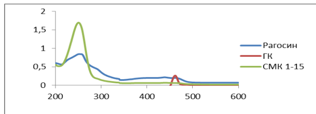
11-rasm. GK:Ragosinni (15:1) nisbatda olingan supramolekular kompleksining UB-spektri
