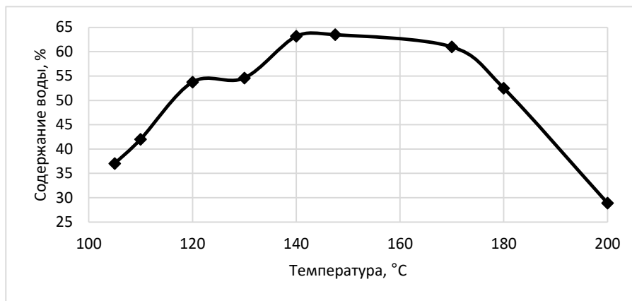
Рис. 2. Количество воды в исследуемых нефтяных шламах
