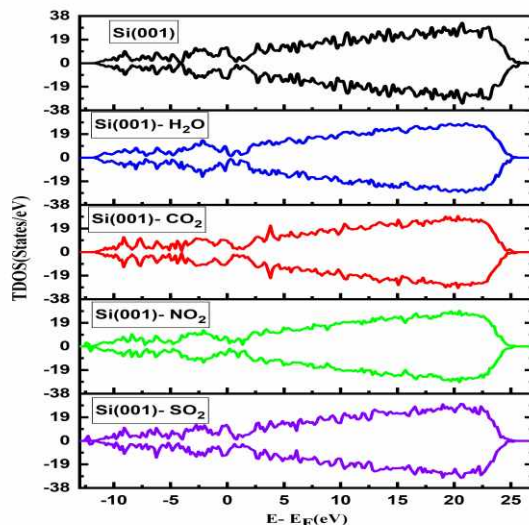
Rasm4. Gaz molekularining Si(001) yuzasida bilan ta'sirlashuvda to'liq elektron holatlar zichligini o'zgarishi(TDOS).
