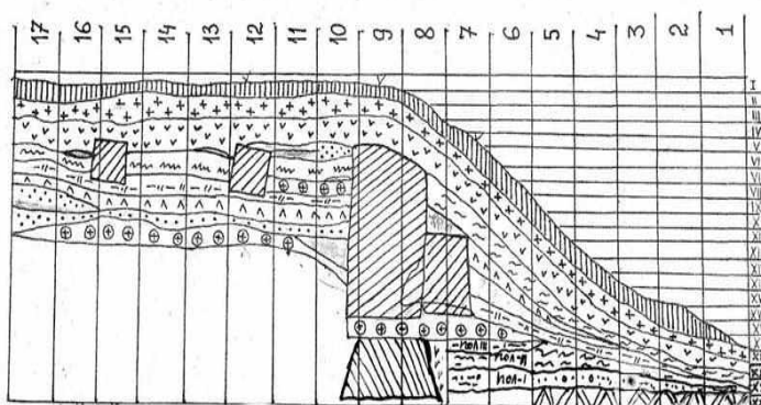
1 - дерновый слой; 2 - глиняные слои; 3 - глиняно-глинистые наклонно залегающие намыты; 4 - глиняно утрамбованная глина прикрытая сверху слоем золы; 5 - наклонная стена; 6 - зола и уголь; 7 - каменная прослойка; 8 - супесчаный слой зеленого и серого цвета; 9 - коричневый мягкий слой; 10 - песок; 11 - серый твердый слой с комками глины; 12 - очаг; 13 - номер помещений.
