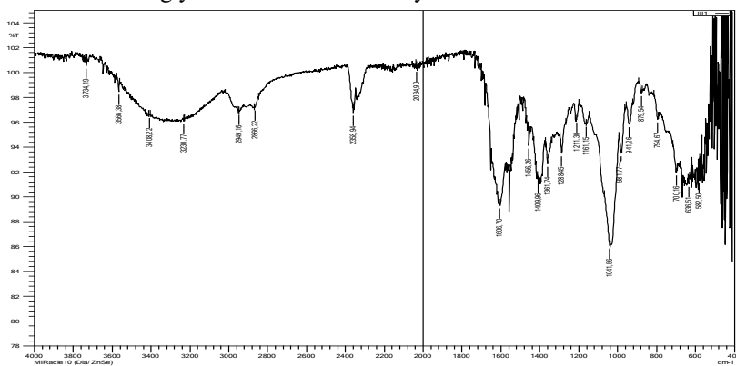
12-rasm. GK:(II) bilan 15:1 supramolekular kompleksi IQ spektri
