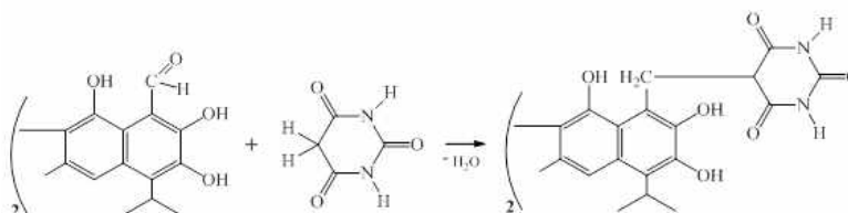
10-rasm: Gossipol moddasining tarkibida metilen guruhi tutgan barbitur kislotasi bilan kondensatsiyalanish reaksiyasi
