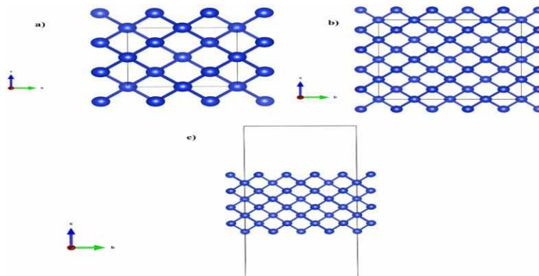
Rasm1. a,b,c Si(001) sirtini hosil qilish ketma-ketligi. a)Kremniy elementar yacheykasi. b)Kremniy superyacheykasi. c)Kremniy sirti
