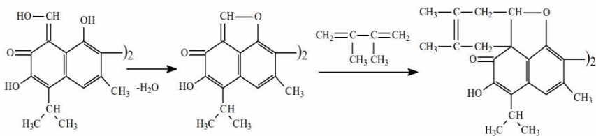
5-rasm: Gossipolning dimetilbutadiyen bilan diyen sintezi reaksiyasi
