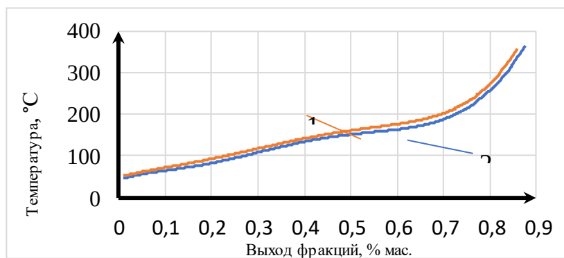
Рис. 3. Итоги экспериментов по изучению фракционного состава смеси нефтегазоконденсата (30% нефти и 70% газоконденсата), проведённых с использованием насадочно-клапанной колонны (2) и клапанной колонны (1).
