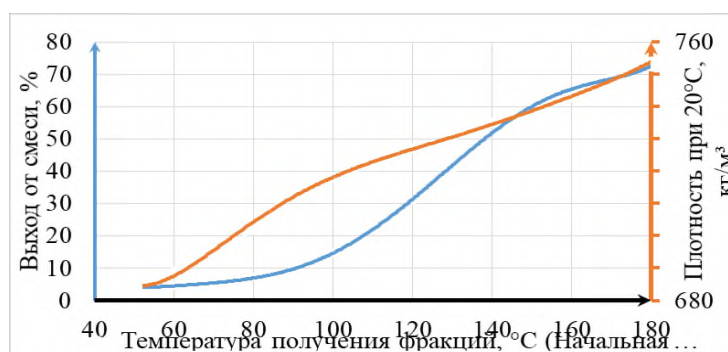
Рис.4. Зависимость выхода и плотности бензиновой фракции от температуры
