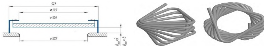
Рис. 1. Сравнительная конструкция элементов колонн: клапанная тарелка и спирально-призматическая насадка 20х30.
