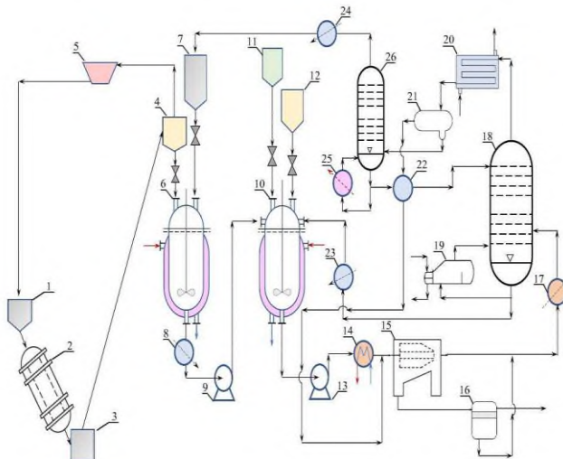
Polipropilen va metilakrilat asosida depressor prisadkalar olish uchun tavsiya etilgan texnologik sxemaning o'ziga xos
