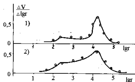
2-сүврет. Өсімлік қалдығы көмірлерінің нәтижелі радиустары бойынша гелек көлемі бөлістіріліуінің дифференциал імек сızıқтары. 1-бойан тамыры қалдығынан алынған көмір, 2-модификацияланған натрий карбонатлы көмір
